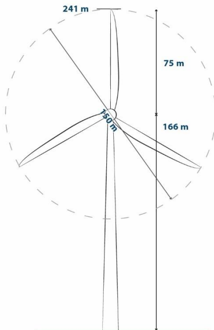
Figuur 29: Belangrijke afmetingen van een windturbine
