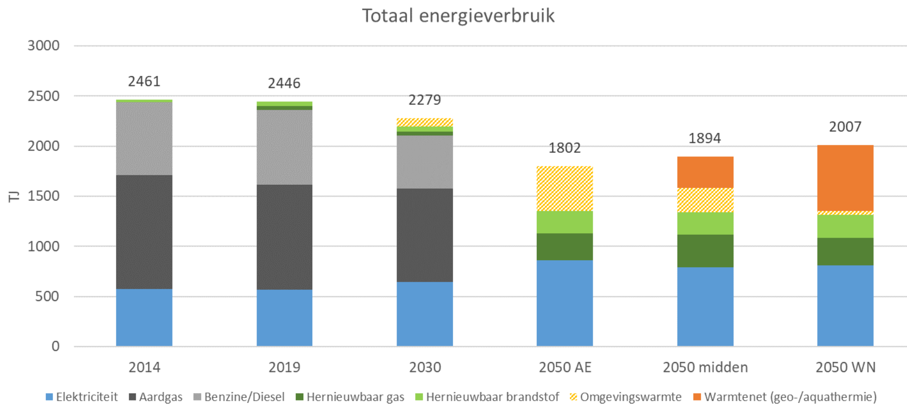
Figuur 28: Overzicht totaal energieverbruik 2014 - 2050 (3 scenario's voor eindsituatie)
