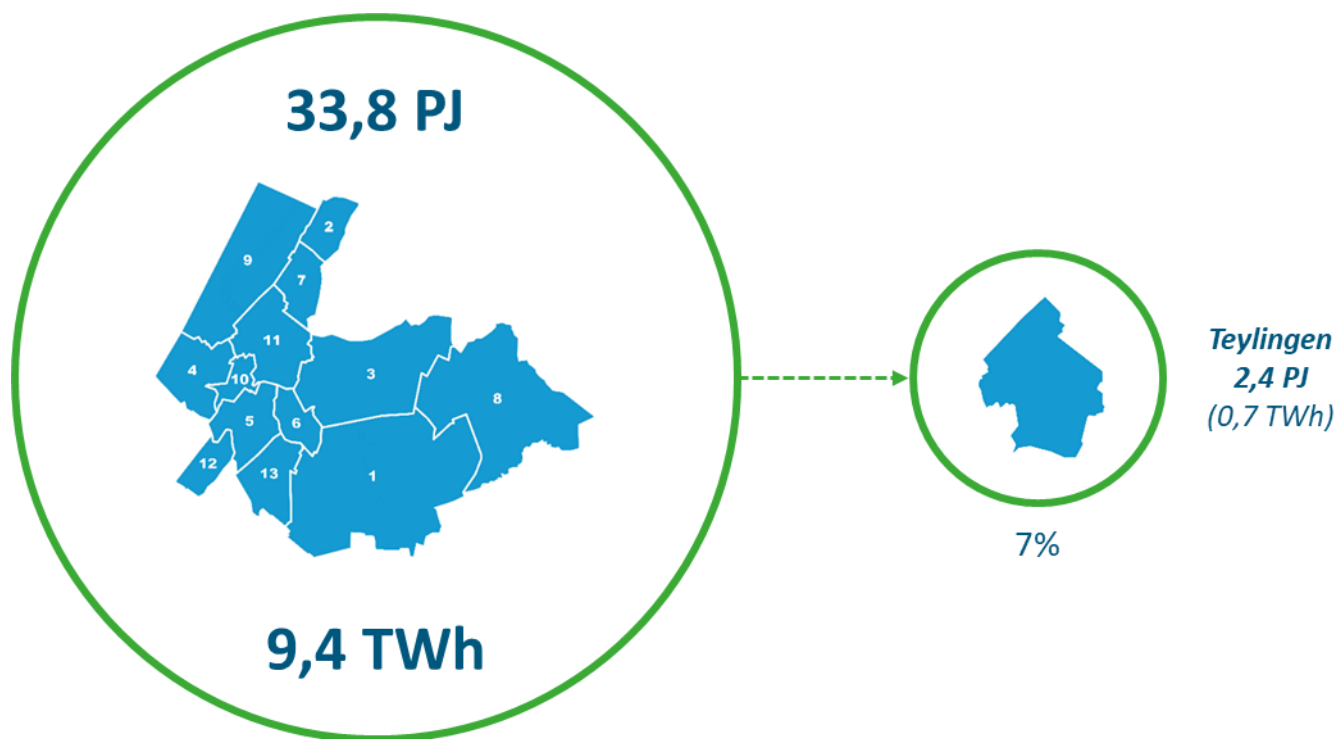
Figuur 6: Totale energieverbruik gemeente Teylingen ten opzichte van totale energieverbruik van Regio Holland Rijnland (2019)
