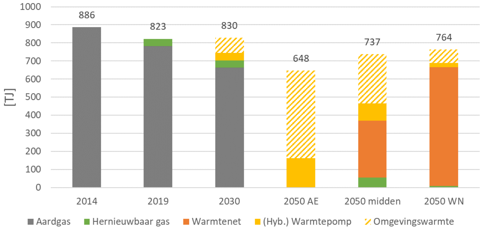
Figuur 27: Warmteverbruik in de gebouwde omgeving. In geel gearceerd is te zien wat het besparingspotentieel is door het toepassen van (hybride) warmtepompen die warmte uit de omgeving (zoals de buitenlucht) gebruiken.
